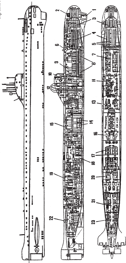
Атомная торпедная подводная лодка пр. 627А («Хит»):
